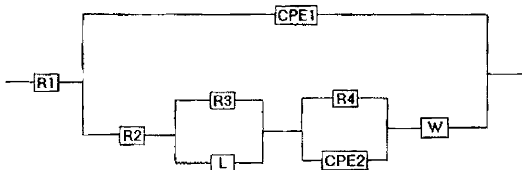
شکل ۸: مدار معادل الکتریکی پیشنهادی برای سیستمهای \text{CuCl-N} و \text{CuCl}_2\text{-N} .
