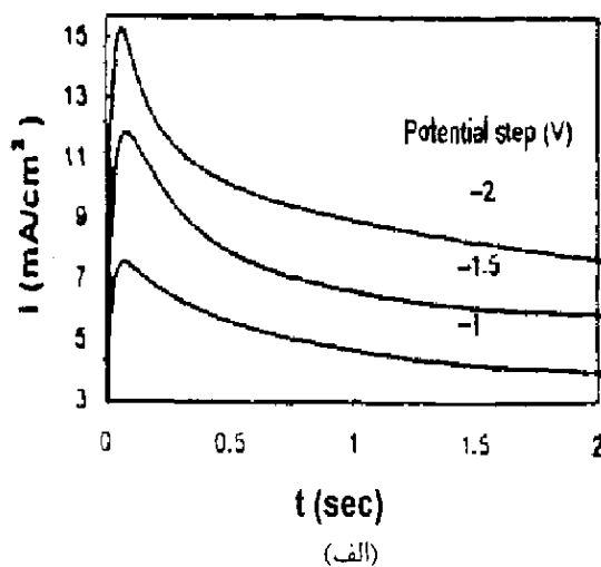
شکل ۵: نتایج آزمایشهای کروئوآمپرومتری در سیستمهای (الف) \text{CuCl}_2\text{-N} و (ب) \text{CuCl-N} .
