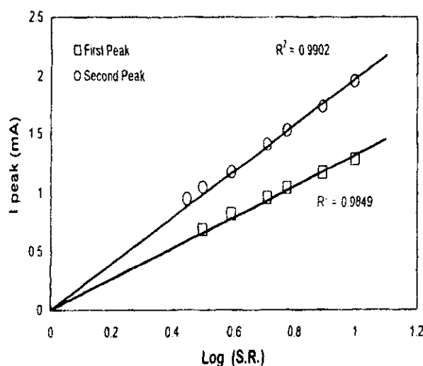
شکل ۳: نمودار تغییرات شدت جریان قله بر حسب جذر سرعت روبش در سیستم \text{CuCl}_2\text{-N} .
